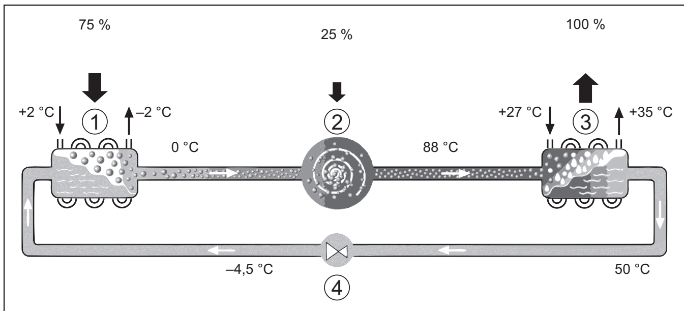
SI.2 Princip delovanja kroga hladilnega sredstva toplotne črpalke
