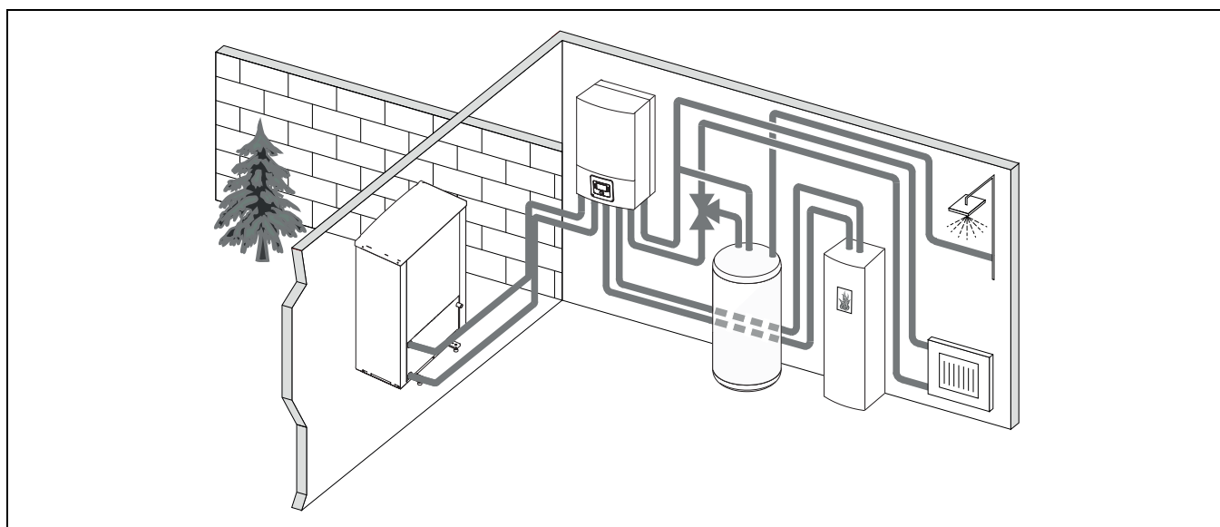
SI.3 Toplotna črpalka Compress 6000 AW, notranja enota AWB brez dodatnega električnega grelnika, zunanji bojler in dodatni zunanji grelnik
