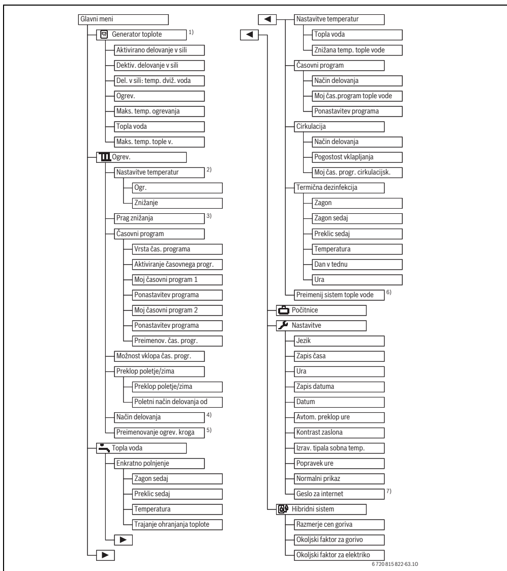
Sl.3 Struktura glavnega menija
