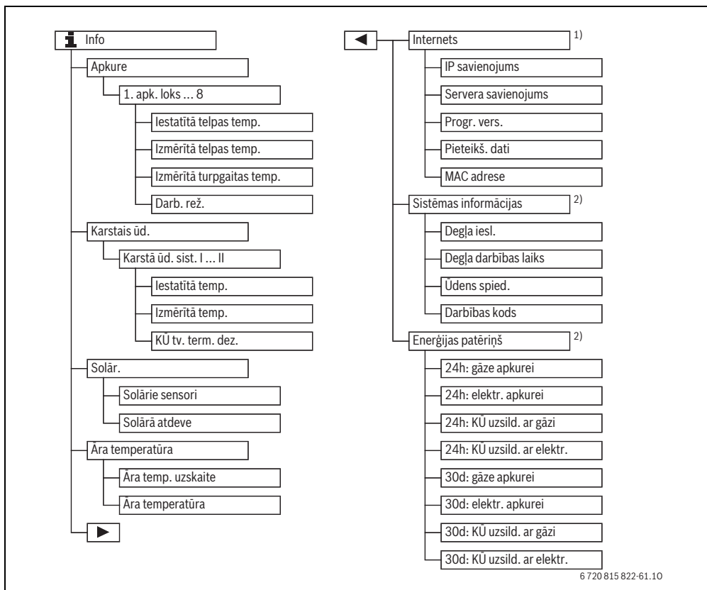
SI.5 Struktūra informacijskega menija
