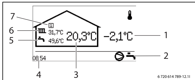
Sl.4 Standardni prikaz
