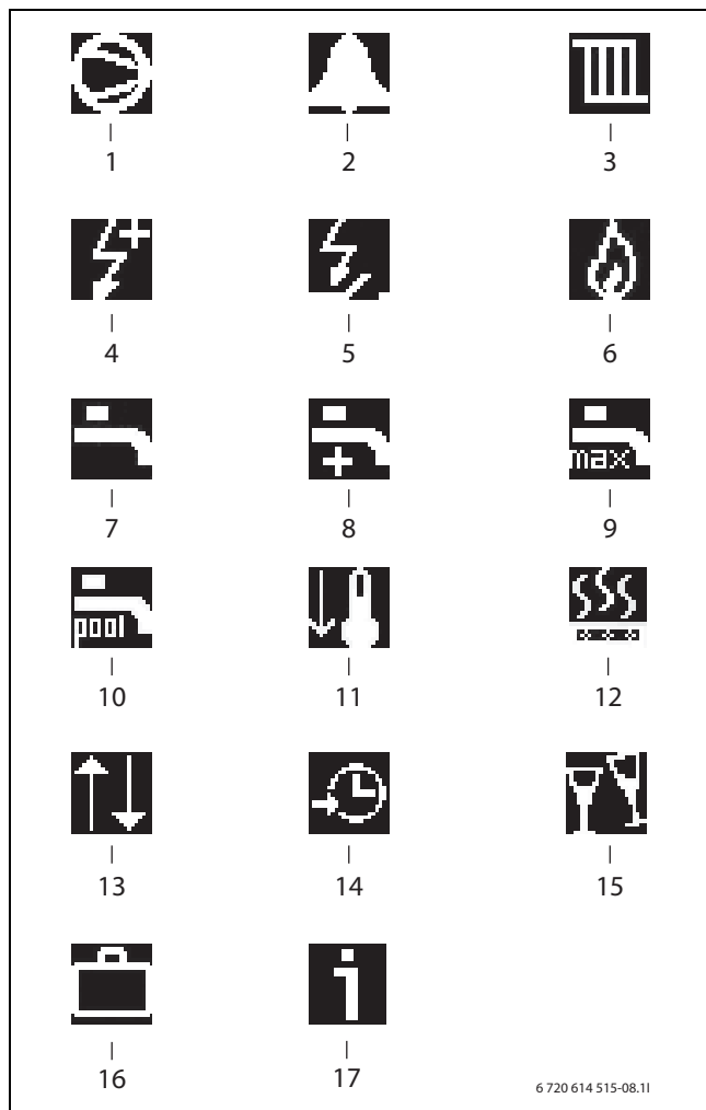
Sl.18 Obratovalni simboli
