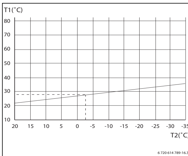
Sl.22 Talno ogrevanje
