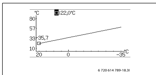
SI.23 Prikaz nastavitve ogrevalne krivulje (ogrevanje)
