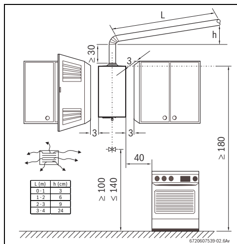
Sl.2 Minimalni odmiki (cm)
