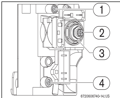
Sl. 15 Točke za merjenje tlaka
