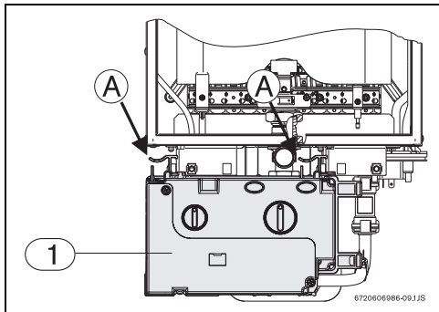
Sl.13 Odstranite nadzorno omarico
