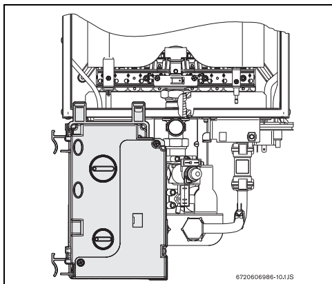
Sl.14 Nadzorna omarica - položaj za uravnavanje plina
