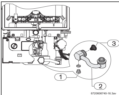
Sl.10 Vijak za izpraznitev
